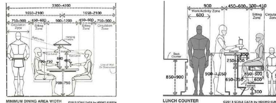
Figura 18: DIMENSIONES ERGONÓMICAS DE CAFETERÍA - RESTAURANTE
