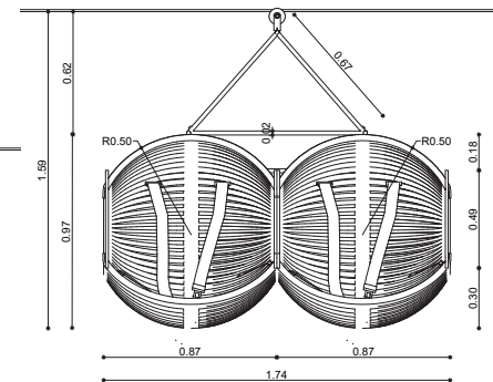
ELEVACION FRONTAL
