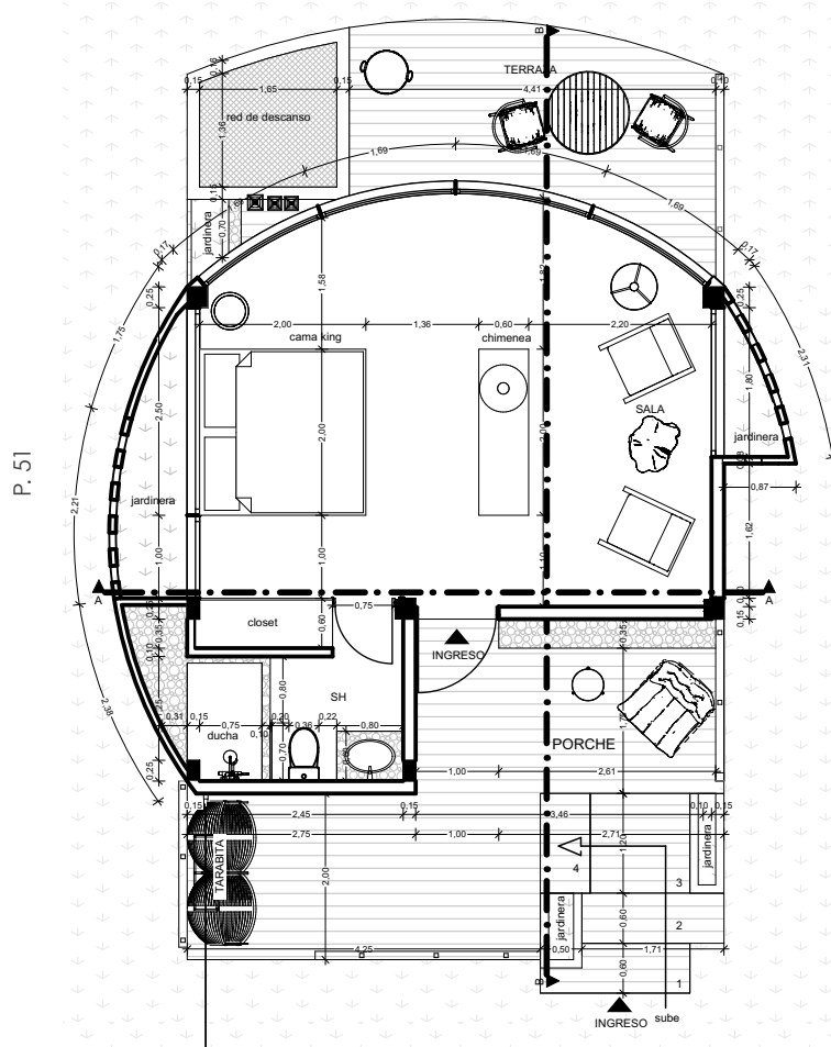
PLANTA ARQUITECTONICA Escala 1:100
