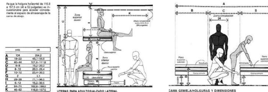
Figura 17: DIMENSIONES ERGONÓMICAS DE HABITACIONES
