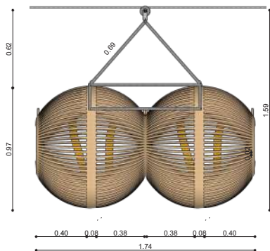
ELEVACION POSTERIOR
