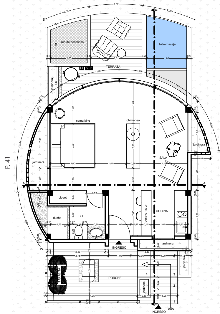
PLANTA ARQUITECTONICA Escala 1:100
