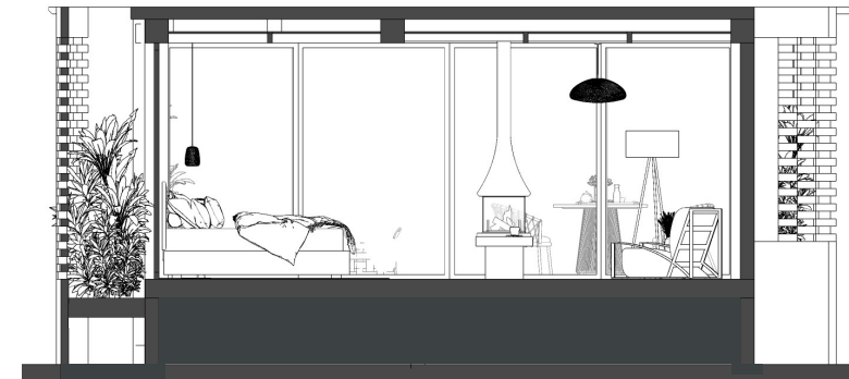
SECCION A-A
