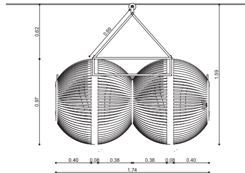
ELEVACION POSTERIOR
