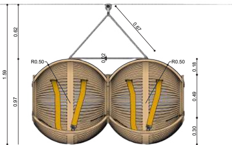
ELEVACION FRONTAL
