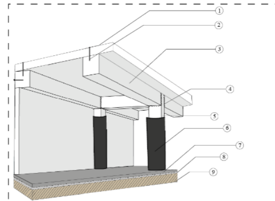
Detalle armado estructura y envoltivo ESC: gráfica
