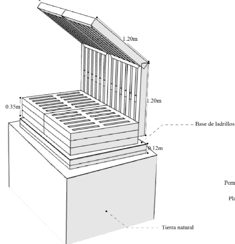
Perspectiva del mobiliario
