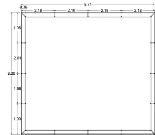
Ubicación planta estructura del contorno de la caja de arena ESC 1:100
