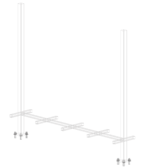
Estructura base del asiento, tubo cuadrado de 50x50x2mm
