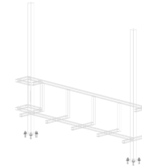
Estructura espaldar y basurero, tubo cuadrado de 50x50x2mm
