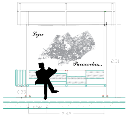
Elevación Frontal ESC 1:75
