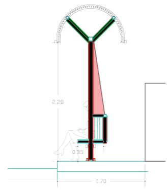
Elevación Lateral ESC 1:75
