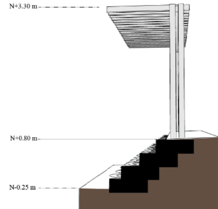
Sección C - C' ESC: gráfica
