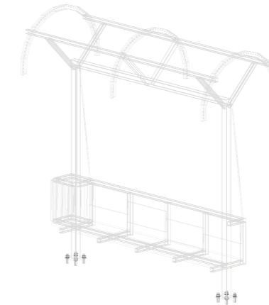
Perfiles transversales de cubierta, tubo circular metálico de 5cm
