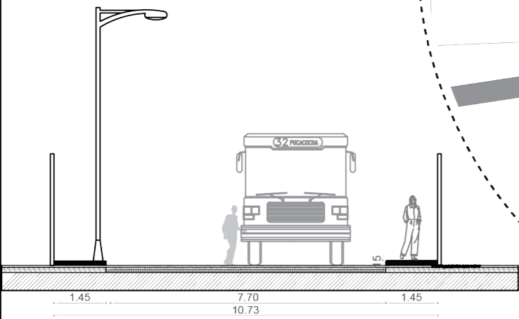
Sección B - B' ESC 1:150
