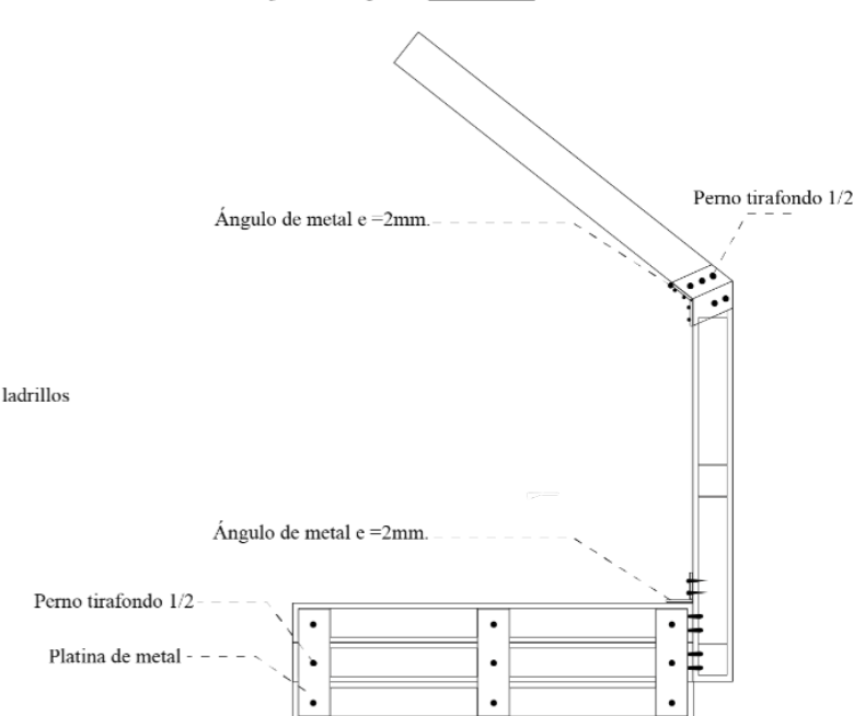
Anclaje de los palets ESC 1: 25
