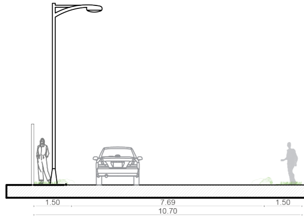
Sección A - A' ESC 1:150
