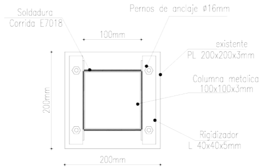
Anclaje ESC 1:75
