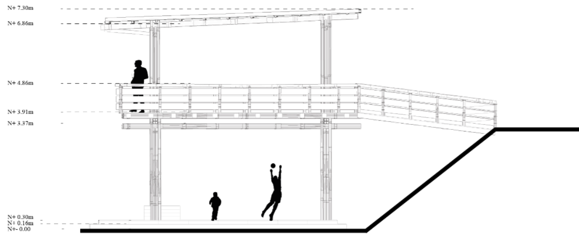
Elevación lateral ESC 1:100
