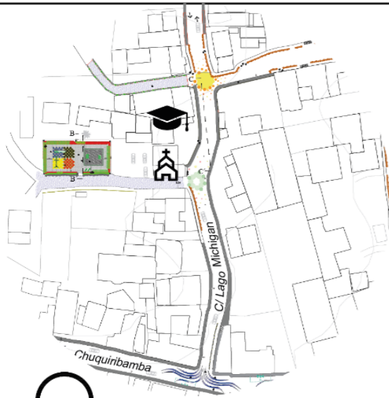
Plano de la Propuesta ESC 1:2500
