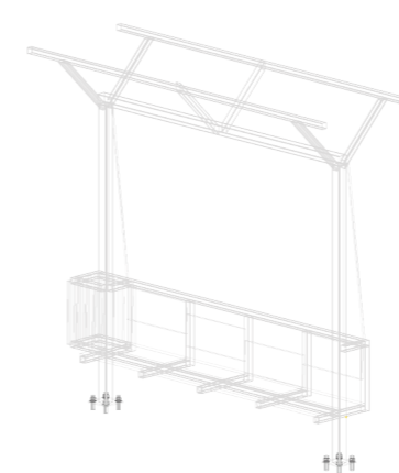
Estructura de cubierta, tubo cuadrado de 50x50x2mm
