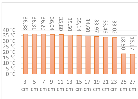
Figura. 13 Datos termómetro infrarrojo LyTrack.
