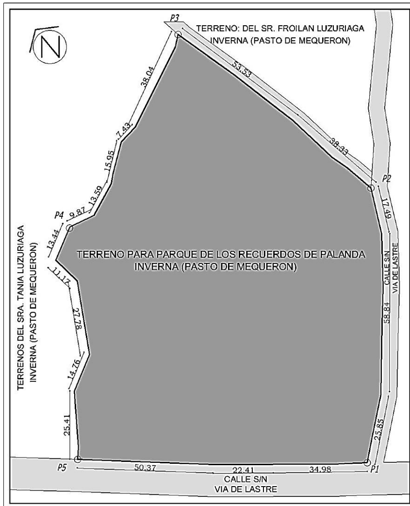
Ilustración 52. Levantamiento del terreno para el nuevo Cementerio en Palanda.
