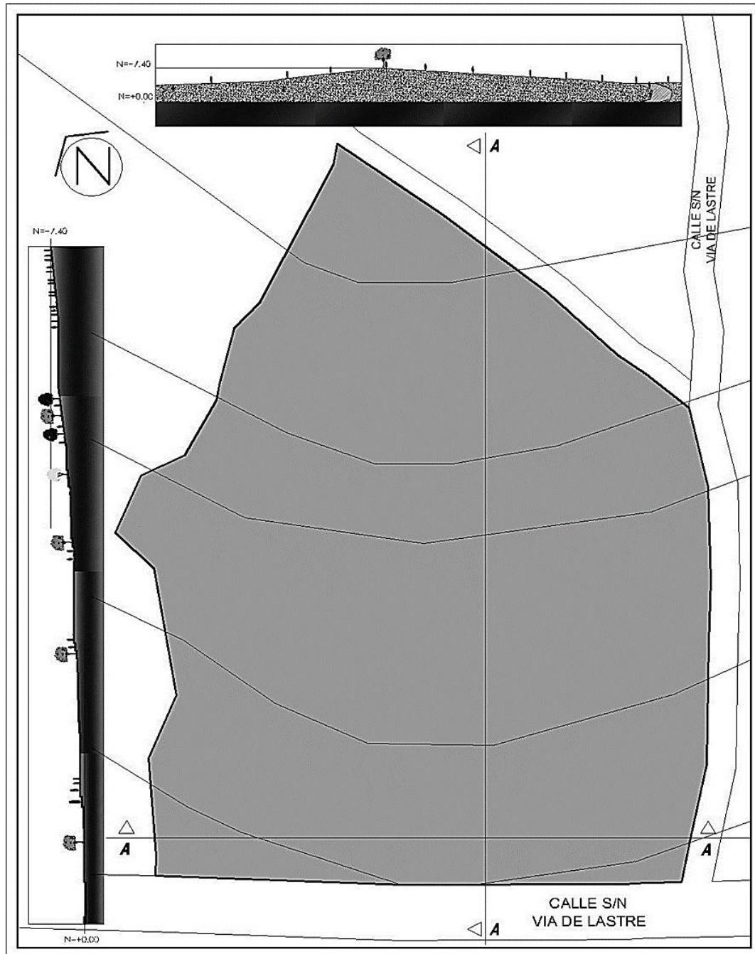
Ilustración 53. Topografía y Cortes del nuevo terreno para el nuevo Cementerio
