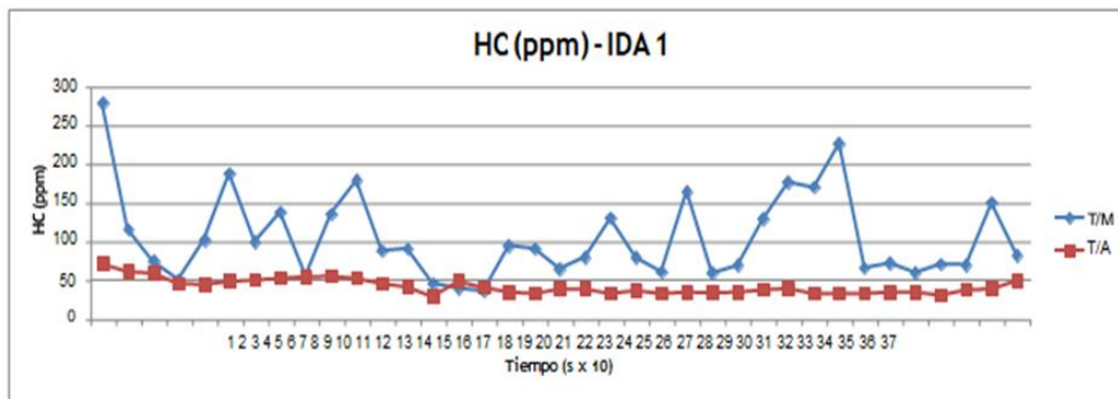
Figura 3. Comparación emisiones de HC en vehículos con transmisión automática y manual
