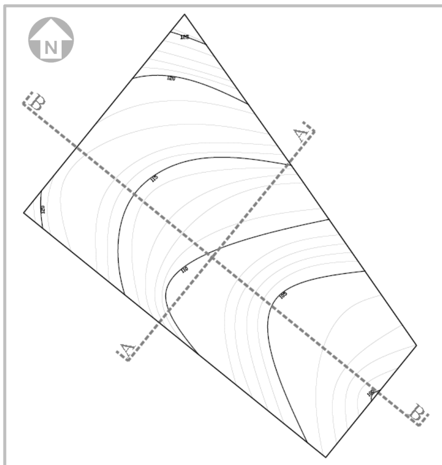
Ilustración 16. Topografía del terreno
