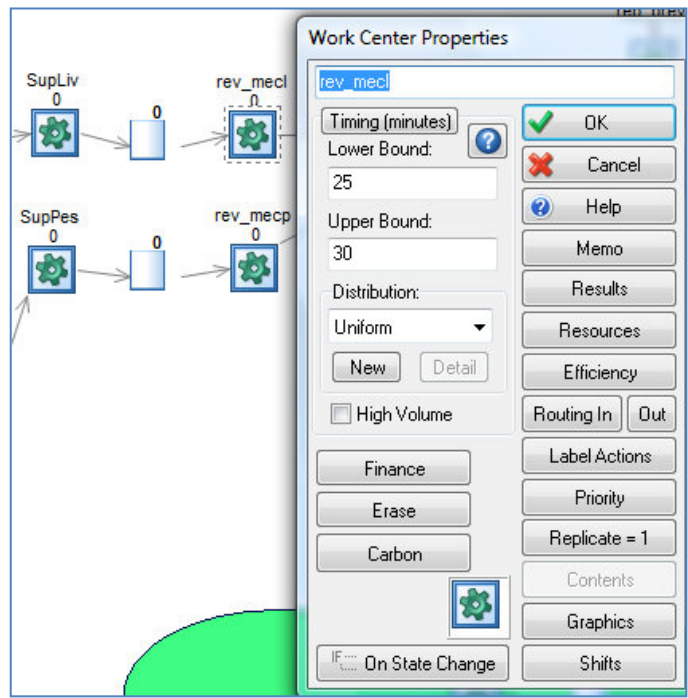
Gráfico N° 28: Propiedades Work Center: revisiones
