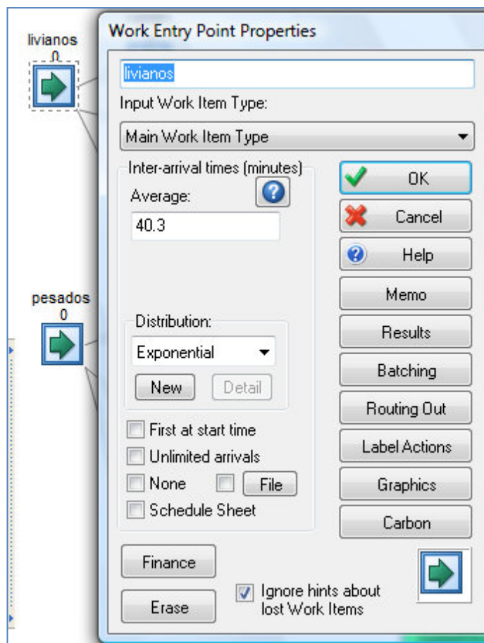
Gráfico N° 26: Propiedades Work Entry Point
