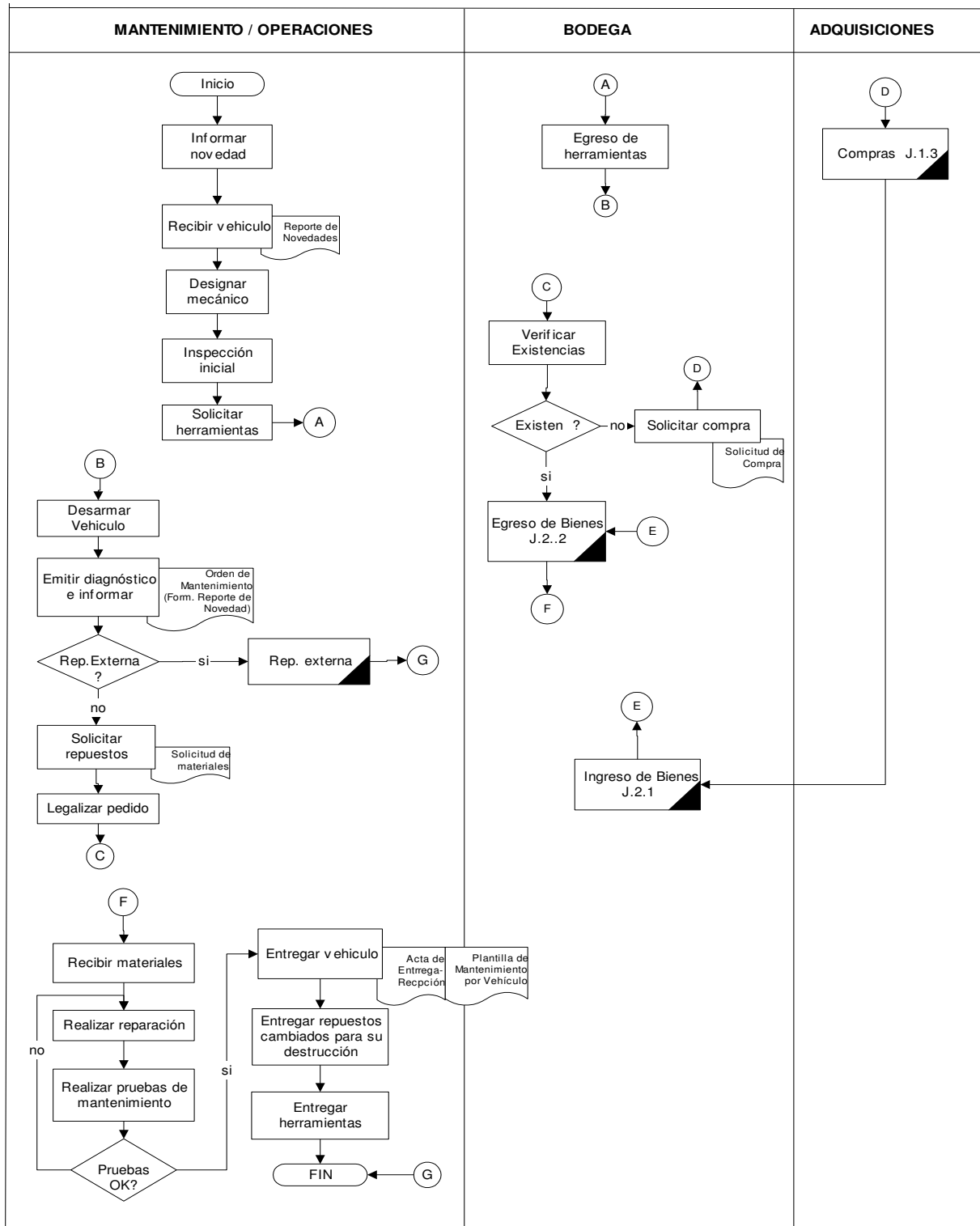
Gráfico N° 45: Diagrama de flujo mantenimiento correctivo.
